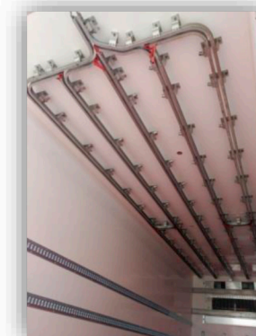
VÍA BIRRAIL
